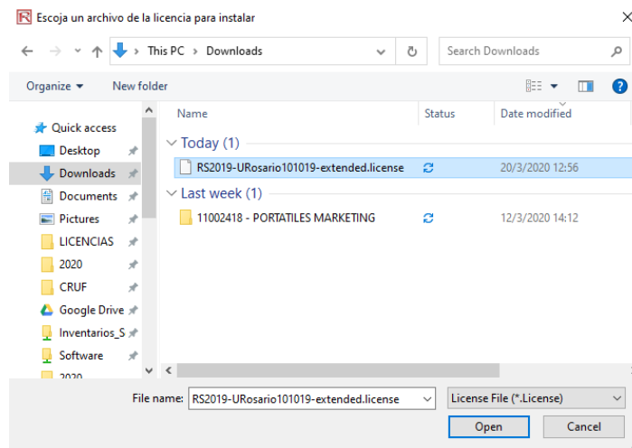
Figura 19. Abrir licencia
