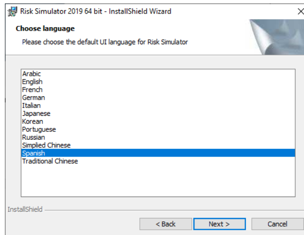
Figura 8. Idioma
