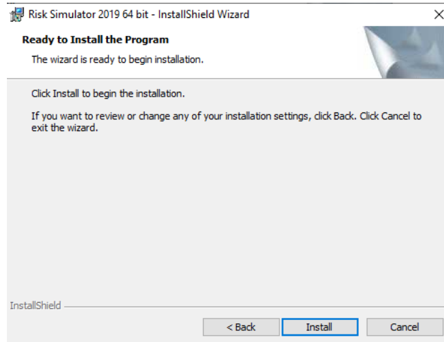
Figura 13. Install
