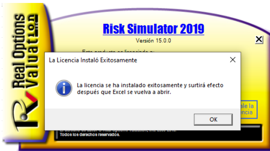
Figura 20. Licencia instalada
