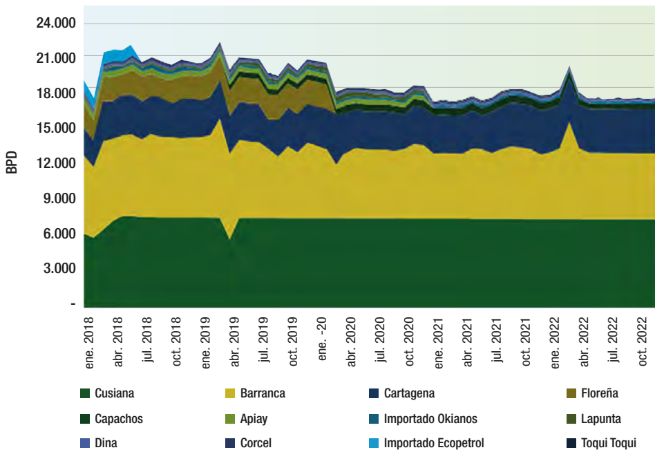
Gráfica 31. Potencial de producción de gas licuado de petróleo mensual por fuente
